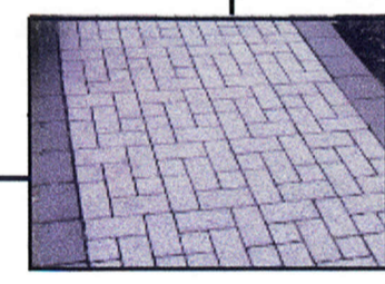
Покрытие из тротуарной плитки типа "брусчатка" (197ммx95ммx60мм)
